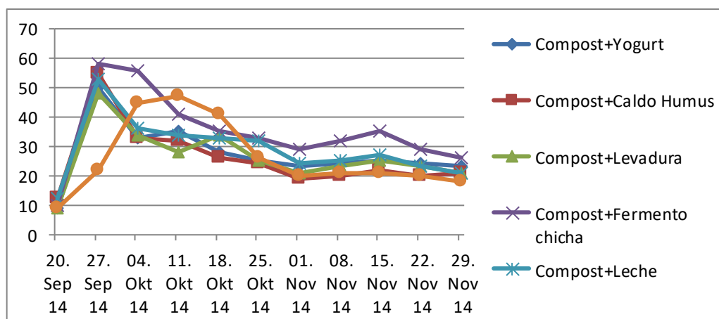
Gráfico 3. Comportamiento térmico del compost durante el período cálido (Septiembre - Diciembre 2014).
