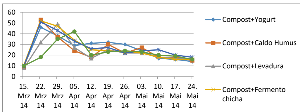
Gráfico 2. Comportamiento térmico del compost durante el período frío (Abril - Junio 2014).
