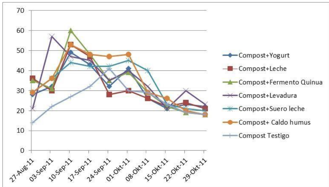
Gráfico 2: Comportamiento térmico durante la compostación a Alto relieve
