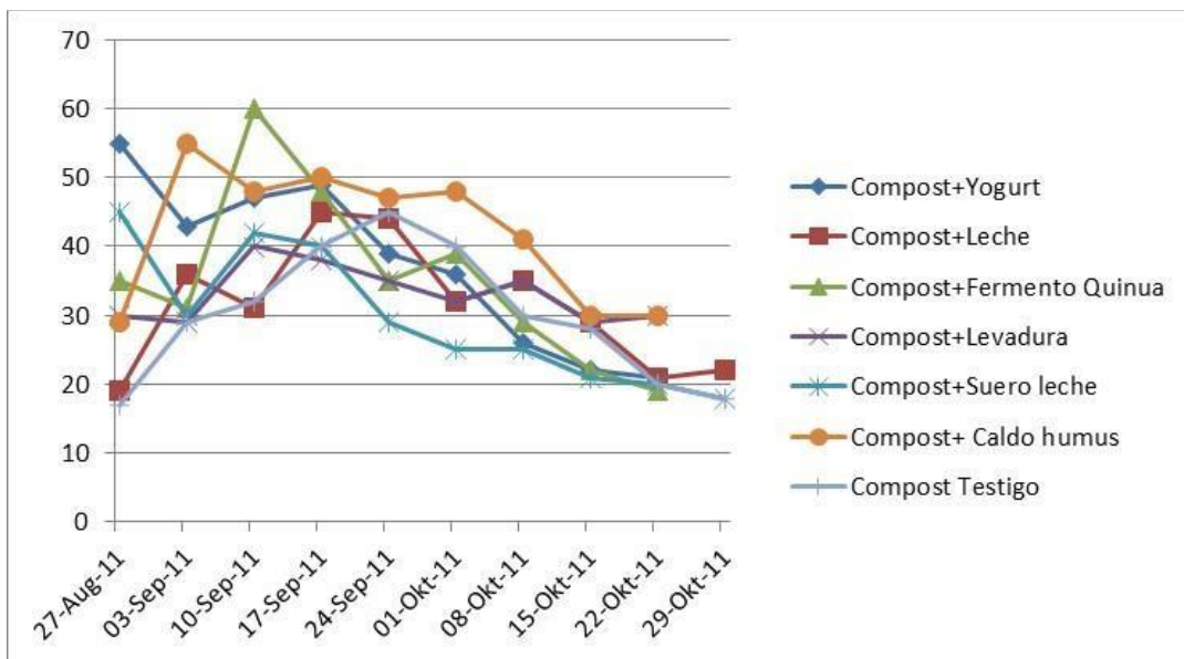
Gráfico 3: Comportamiento térmico durante la compostación a Bajo relieve
